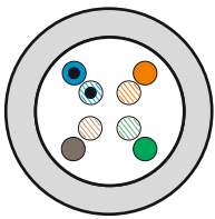
Průřez kabelem MODnet
